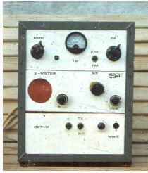
2m AM/FM Sender /Empfänger mit QOE03/12 und EL34 im Modulator, OE7IW
