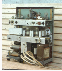
Rückansicht des OE7IW Gerätes, Nuvisor 2m Tuner in den 50-60er Jahren
