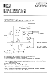
Anschlussvorschlag VFO
