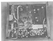
Bild 96. Innenaussicht des 70cm-Zusatzgerätes von DL 6 MH.
