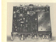
Bild 88. Innenansicht der 2-m-Station von DL9AL
