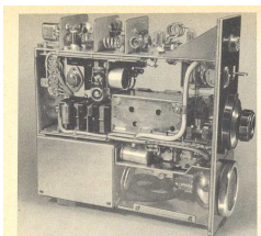
Bild 87. 2-m-Station von DL 9 AL, Innenansicht von der Tuner-Seite
