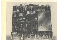
Bild 88. Innenansicht der 2-m-Station von DL 9 AL
