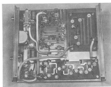
Bild 95. Innenansicht des 70cm-Zusatzgerätes von DL 6 MH.
