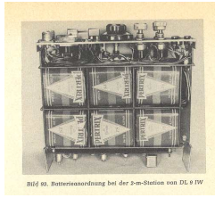
Bild 90. Batterieanordnung bei der 2-m-Station von DL 9 IW
