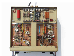
Radio-Bitter Minitix UKS3
