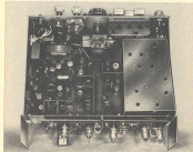
Bild 20. Innensicht der 2-m-Station von DL 9 IW
