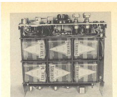
Bild 21. Batterieanordnung bei der 2-m-Station von DL 9 IW
