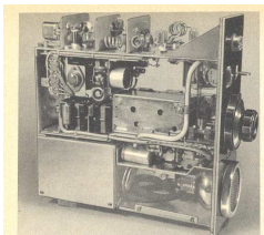
Bild 87. 2-m-Station von DL9AL. Innensicht von der Tuner-Seite
