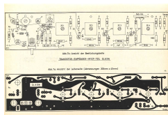
Empfänger Leiterplatte
