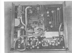
Bild 92. Innenansicht des 70cm-Zusatzerzeugnis von DL 6 MH.
