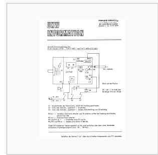
Anschlussvorschlag VFO
