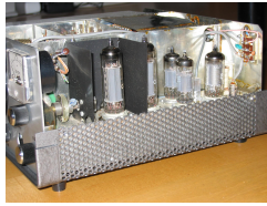
Detailansicht der Endstufe
