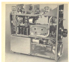
Bild 67. 2m-Station von DL9AL, Innenansicht von der Tuner-Seite
