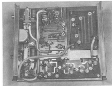
Bild 92: Innensicht des 70-cm-Zusatzgerätes von DL 6 MH.
