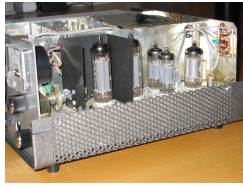
Detailansicht der Endstufe
