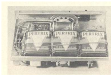
Bild 63. Unterbringung der Batterien unter dem Chassis
