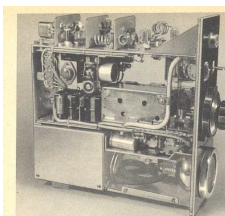
Bild 67. 2-m-Station von DL9AL, Innenansicht von der Tuner-Seite
