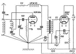
Audionsschaltung
