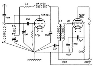
Audionsschaltung
