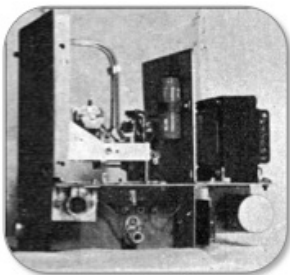
Wallmann Konverter Seitenansicht
