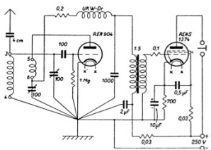
Audionsschaltung
