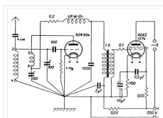
Audionsschaltung
