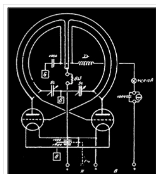
Gegentaktsender
