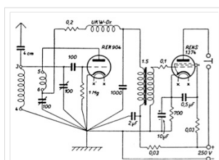
Audionsschaltung
