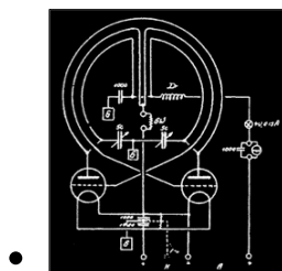
Gegentaktsender
