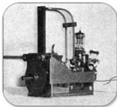
Wallmann Konverter: Oszillator
