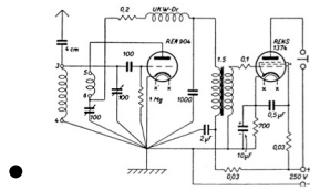
Audionsschaltung
