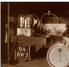
Sender Rudi Rapcke, Kurzwellentechnik des DASD 1935
