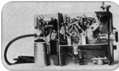
Richard Auerbach, DL1FK: Ansicht von unten
