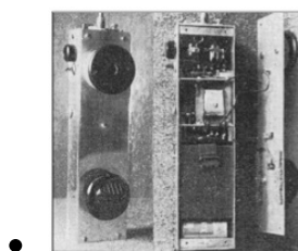
2m Transceiver (Handfunksprechgerät) aus CQ 10/1949 von Bernd Cramer, DL3XC
