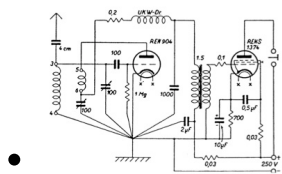
Audionsschaltung
