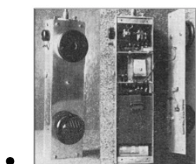
2m Transceiver (Handfunksprechgerät) aus CQ 10/1949 von Bernd Cramer, DL3XC
