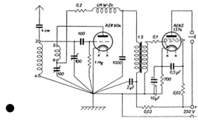
Audionsschaltung
