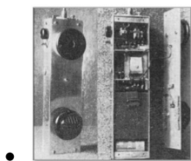
Gegentaktsender
