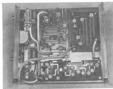
Bild 92. Innensicht des 70cm-Zusatzgerätes von DL 6 MH.
