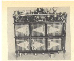
Bild 60. Batterieanordnung bei der 3-m-Station von DL 9 IW
