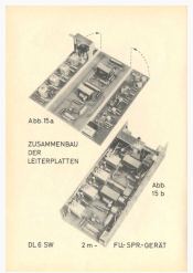
Zusammenbau Leiterplatten
