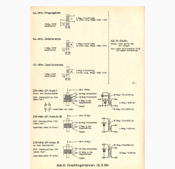
Empfängerspulen
