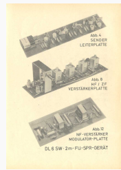
Leiterplatten Abb.
