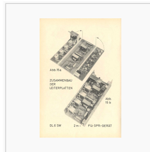
Zusammenbau Leiterplatten
