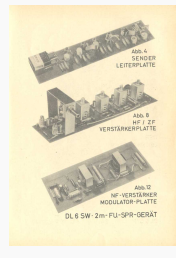
Leiterplatten Abb.
