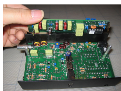
Einbau Antennentuner
