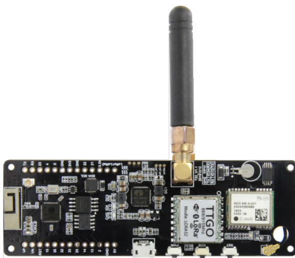
LILLYGO-TTGO-LoRa-Modul
