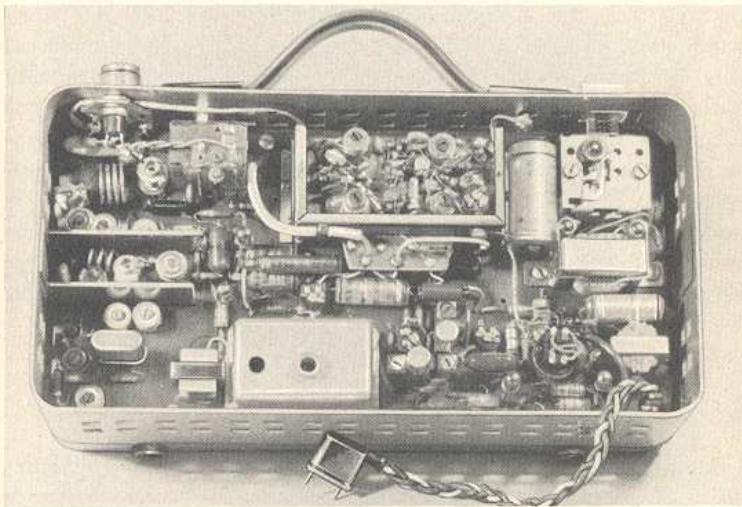
Bild 88. Innenansicht der kleinen Transistorstation von DL 9 AL
