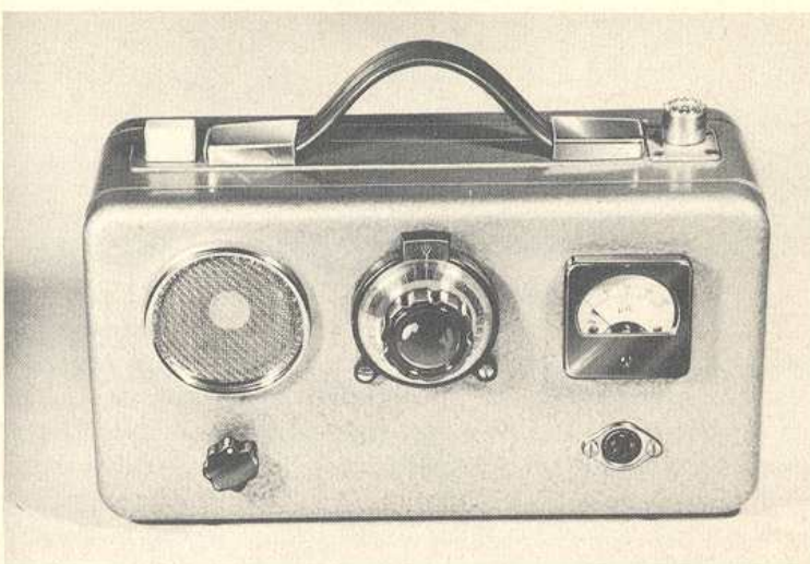
Bild 87. Frontansicht einer kleinen Transistorstation von DL 9 AL
