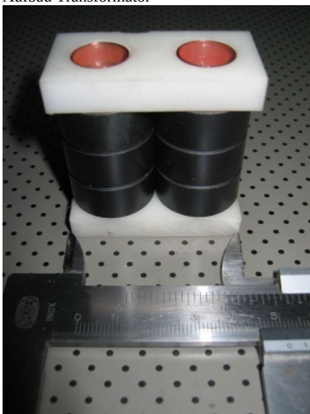
Aufbau Transformator
