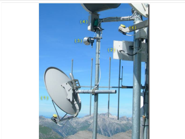
OE7XLT Empfangsantennen
