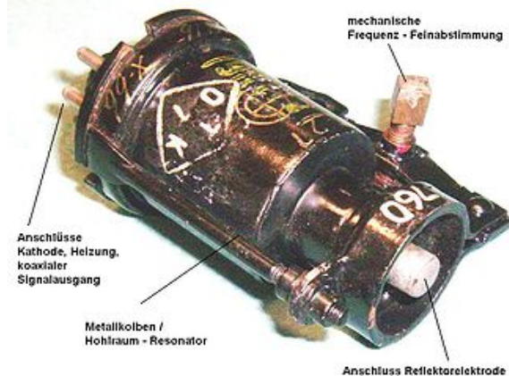
Prinzipaufbau des Klystrons
