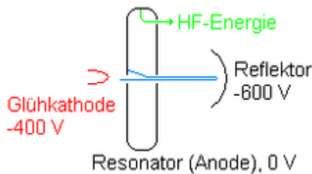
Prinzipaufbau des Klystrons
