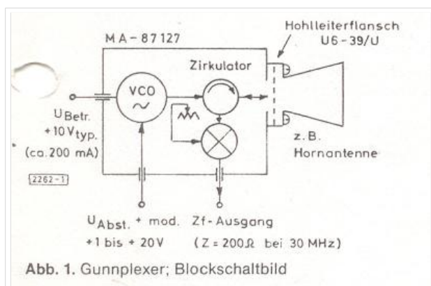
Blockschaltbild MA87127
