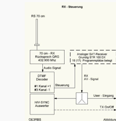
RX Steuerung
