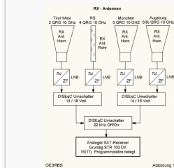
RX Antennen
