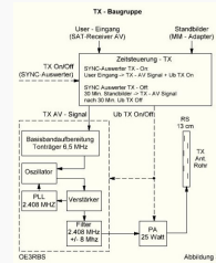
TX Baugruppe
