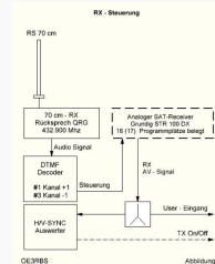
RX Steuerung
