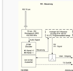
RX Steuerung
