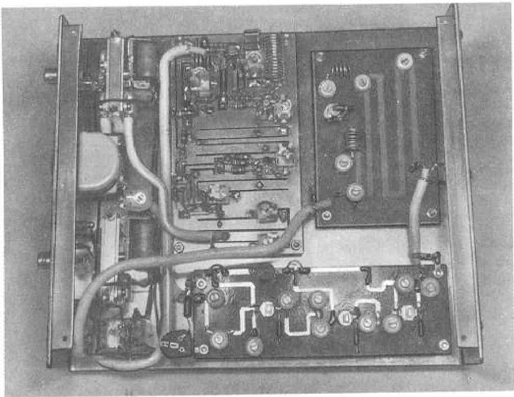
Bild 92. Innenansicht des 70-cm-Zusatzgerätes von DL 6 MH.
