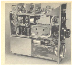
Bild 89. 2-m-Station von DL 9 AL, Innensicht von der Tuner-Seite
