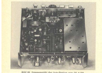
Bild 90. Innensicht der 2-m-Station von DL 9 AL
