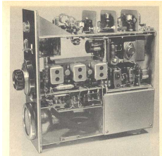
Bild 88. Innensicht der 2-m-Station von DL 9 AL mit Zf-Baustein
