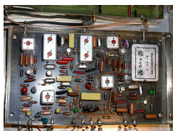
ZFB9/02 9MHZ IF- Amplifier
