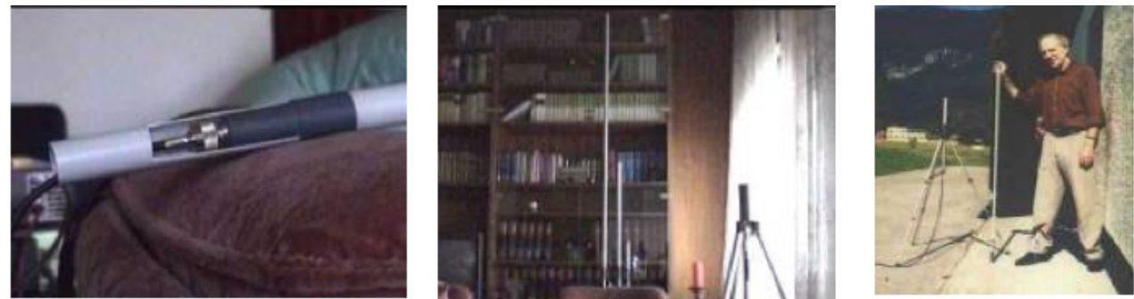
Schnitt Antennenfuß mit Mastrohr Baugrößenvergleich 80m/40m/10m Der Verfasser mit 80m System, auf Stativ 10m System Es ist keine höhere Auflösung vorhanden.
