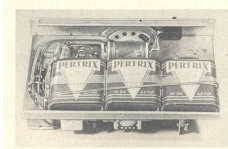
Bild 81. Unterbringung der Batterien unter dem Chassis
