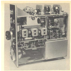
Bild 88. Innenaussicht der 2-m-Station von DL9AL mit ZF-Baustein
