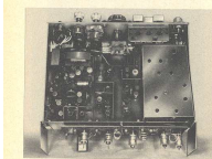
Bild 90. Innenaussicht der 2-m-Station von DL9AL
