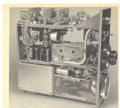
Bild 47. 2-m-Station von DL 9 AL, Innenansicht von der Tuner-Seite
