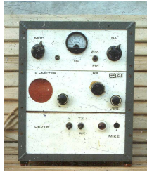
2m AM/FM Sender /Empfänger mit QJE03 /12 und EL34 im Modulator, OE7IW
