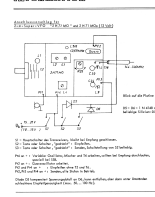
Anschlussvorschlag VFO
