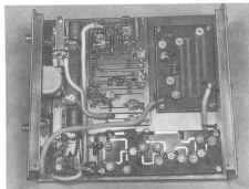
Bild 92. Innenaussicht des 70cm-Zustückgerätes von DL 6 MH.
