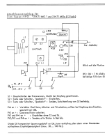
Anschlussvorschlag VFO
