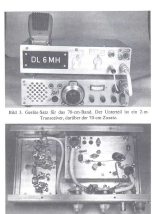
Bild 94. Innenaussicht des in Bild 3 gezeigten 'Trans-Duplex-Converters'. Links der Frequenzumwandler, rechts der Transceiver nach DL 6 MH.
