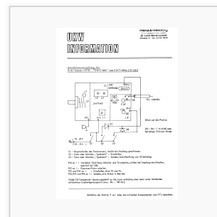
Anschlussvorschlag VFO
