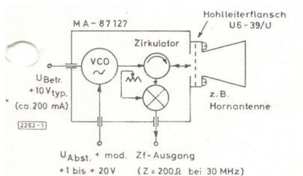
Abb. 1. Gunnplexer; Blockschaltbild
